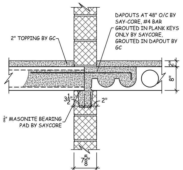
TYP. SECTION
