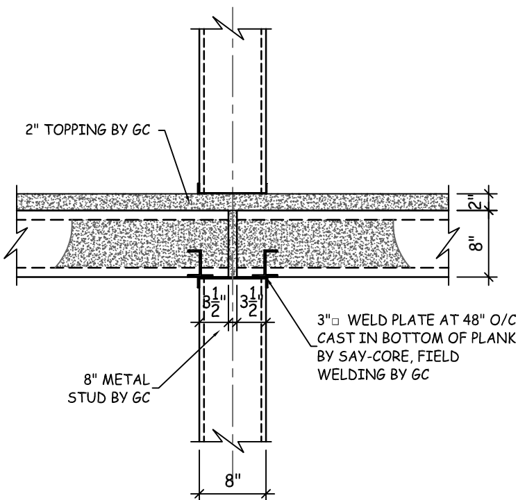
TYP. SECTION
