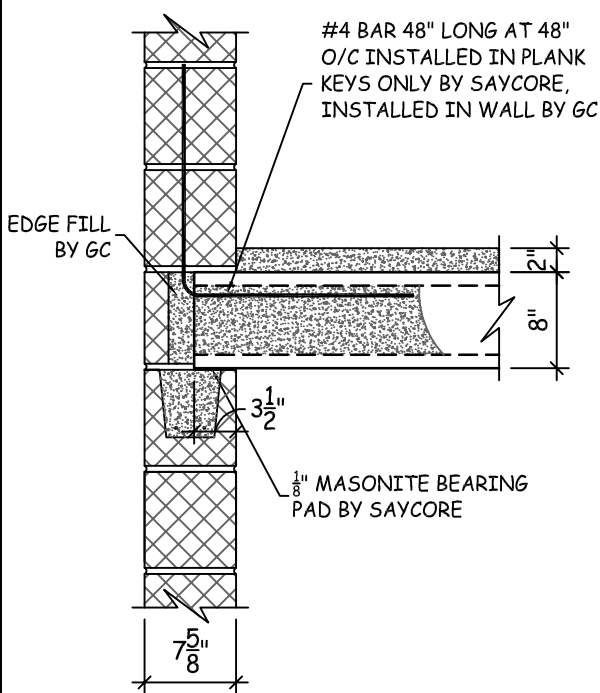
TYP. SECTION
